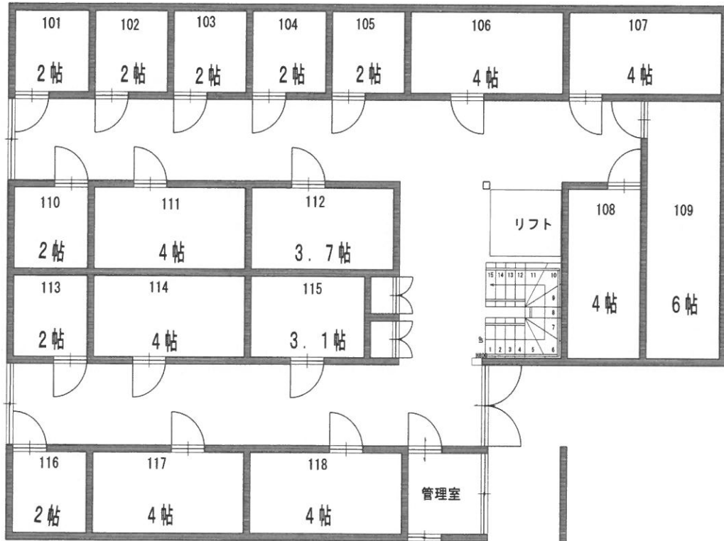
1階間取図
